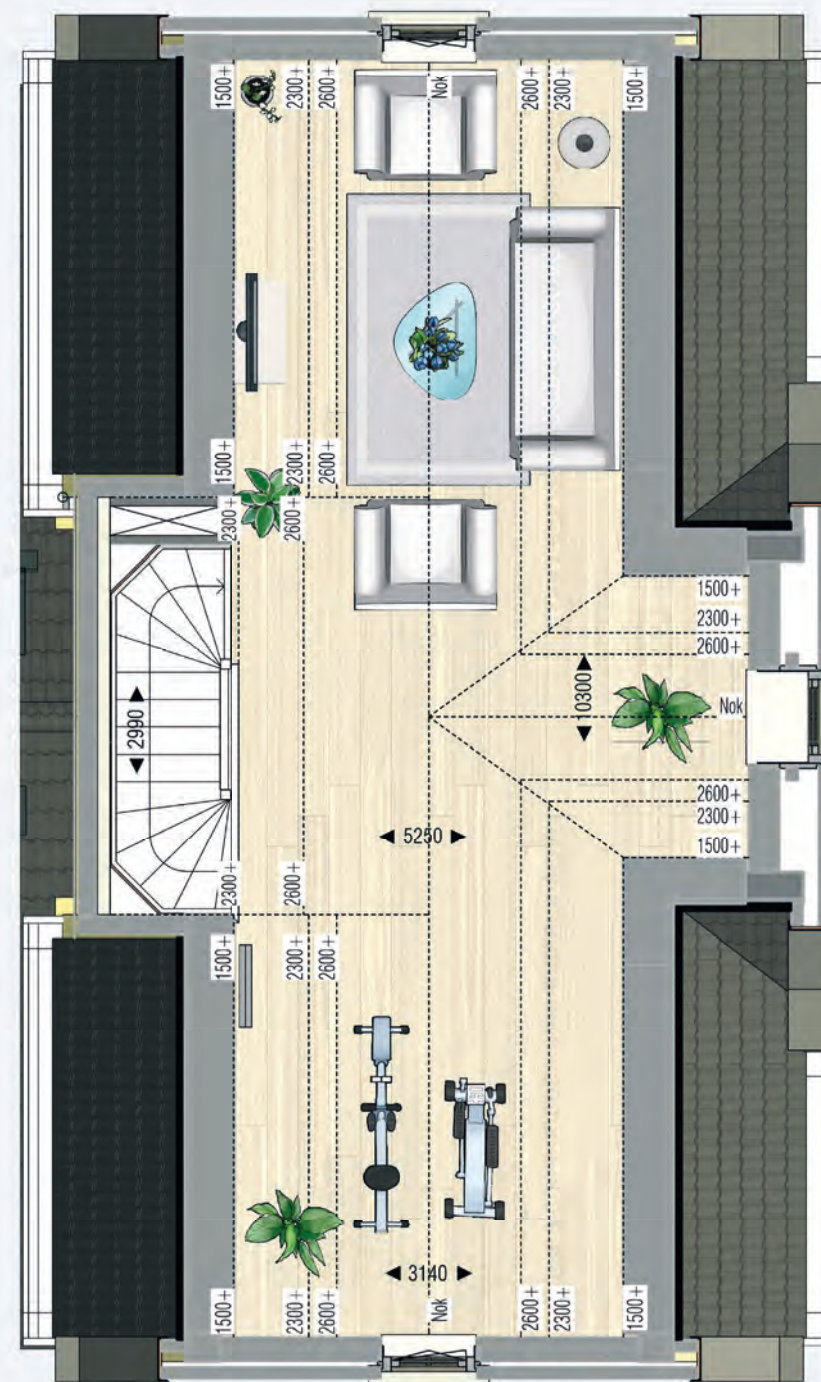
Parkzicht 27 (standaard dakkappel), 33, 60, 67.
